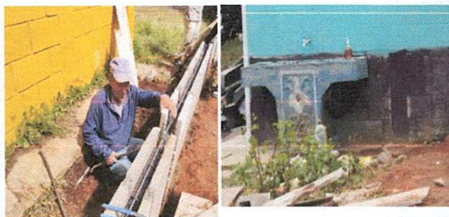
Foto 4: Mejoramiento de drenaje y muro perimetral
